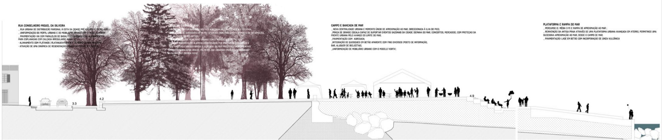
CAMPO DE MAR, BANCADA E RAMPA DO CANAL DO FAIAL . CORTE TRANSVERSAL 1:200
