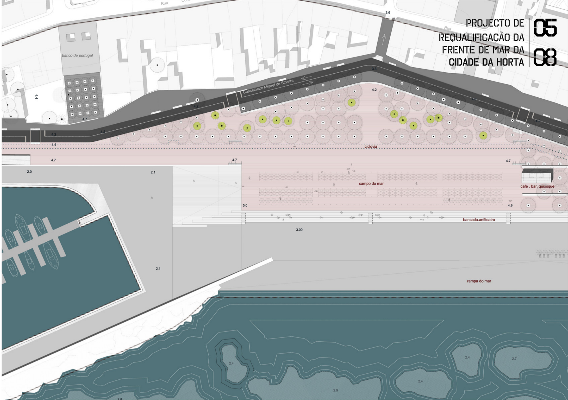
A3. CAMPO DE MAR E RAMPA DO CANAL FAIAL E PASSEIO MARÍTIMO 1:500
